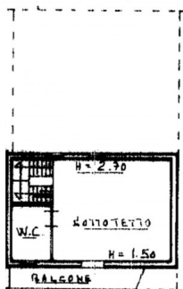
SECONDO PIANO
