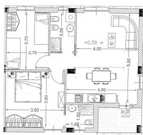
PIANTA VILLA 2
