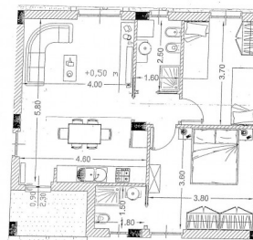
PIANTA VILLA 1
